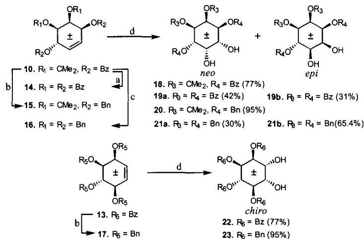
Scheme 2. Reagents and conditions: a. i) 80% aq. AcOH, 100 °C, ii) BzCl, pyridine, 91%; b. i) NaOMe, MeOH, ↑↓, ii) BnBr, NaH, DMF, 90-95%; c. i) 80% aq. AcOH, 100 °C, ii) NaOMe, MeOH, ↑↓, iii) BnBr, NaH, DMF, 87%; d. OsO 4 , NMO, aq. acetone.
